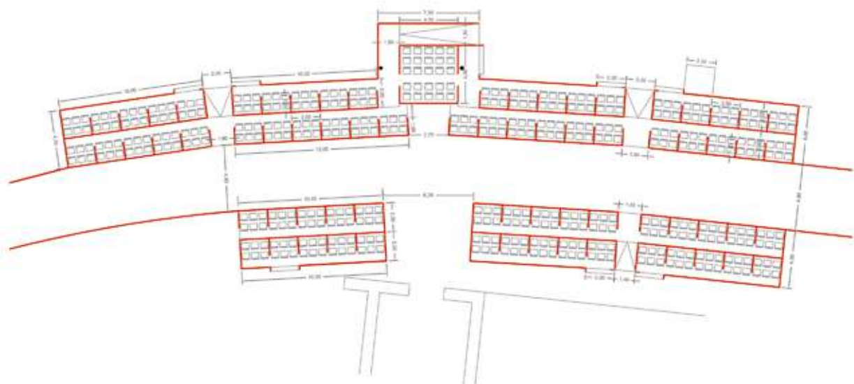
PROYECTO PARA LA NUEVA UBICACIÓN DE LA TRIBUNA DE SEMANA SANTA DE VÉLEZ-MÁLAGA AGRUPACIÓN DE COFRADÍAS DE SEMANA SANTA DE VÉLEZ-MÁLAGA PLANO DE PLANTA. Fase I Febrero-2016
